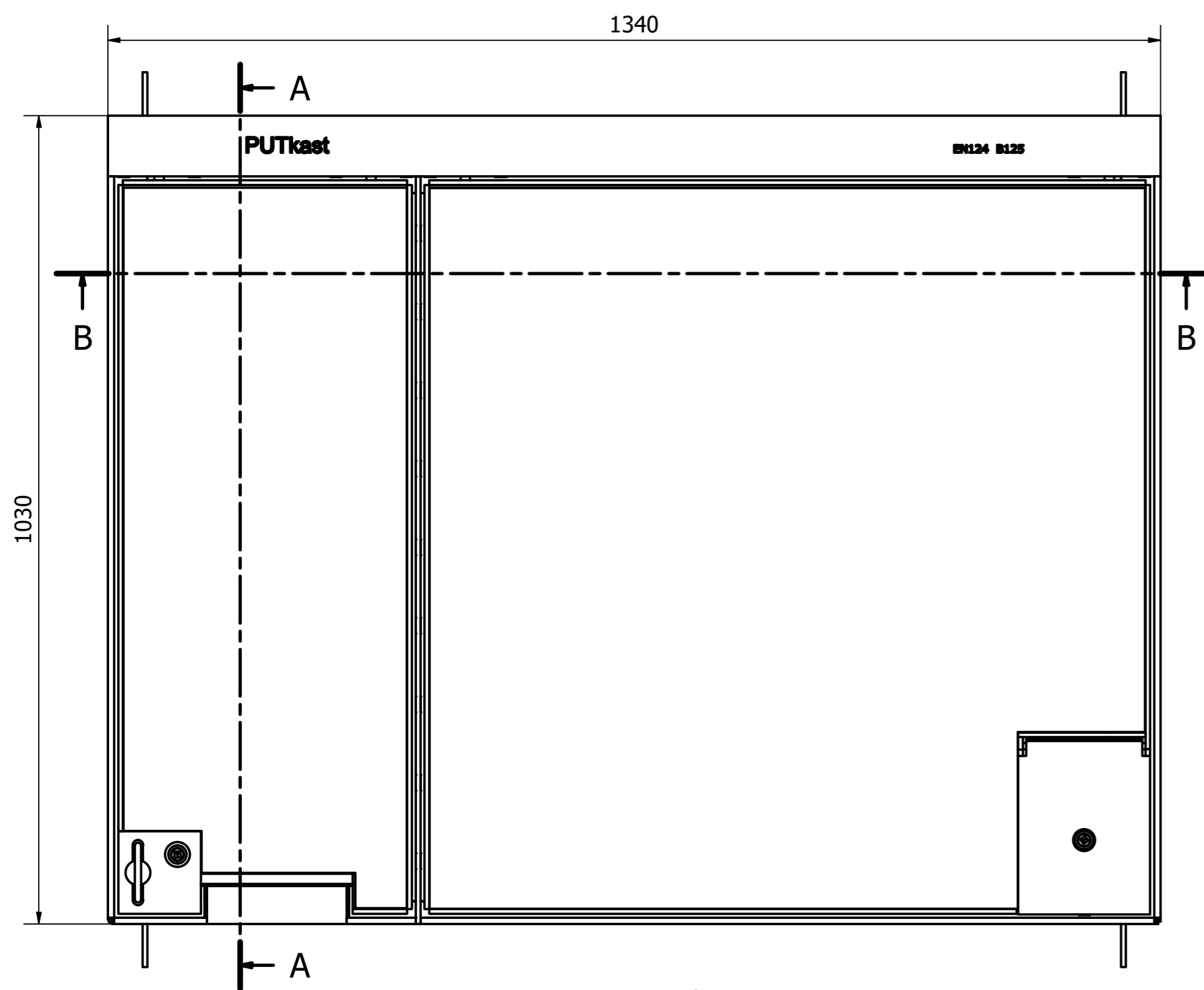
Bovenaanzicht
