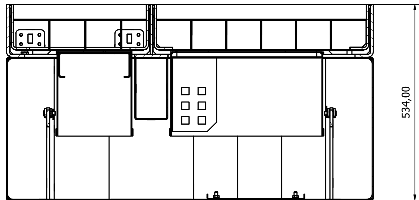
Vooraanzicht : B-B ( 1 : 6 )
