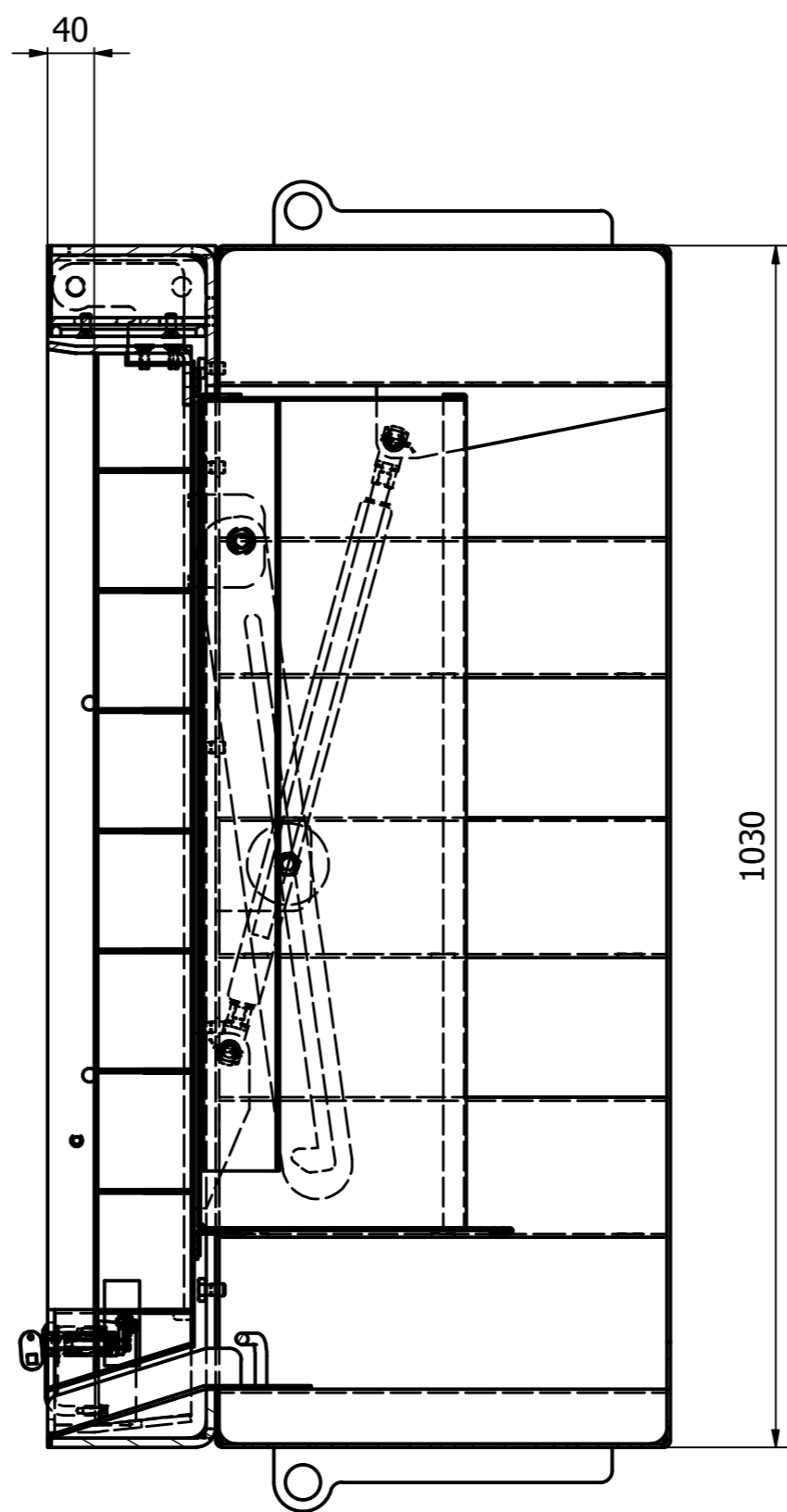
Rechterzijaanzicht : A-A ( 1 : 6 )
