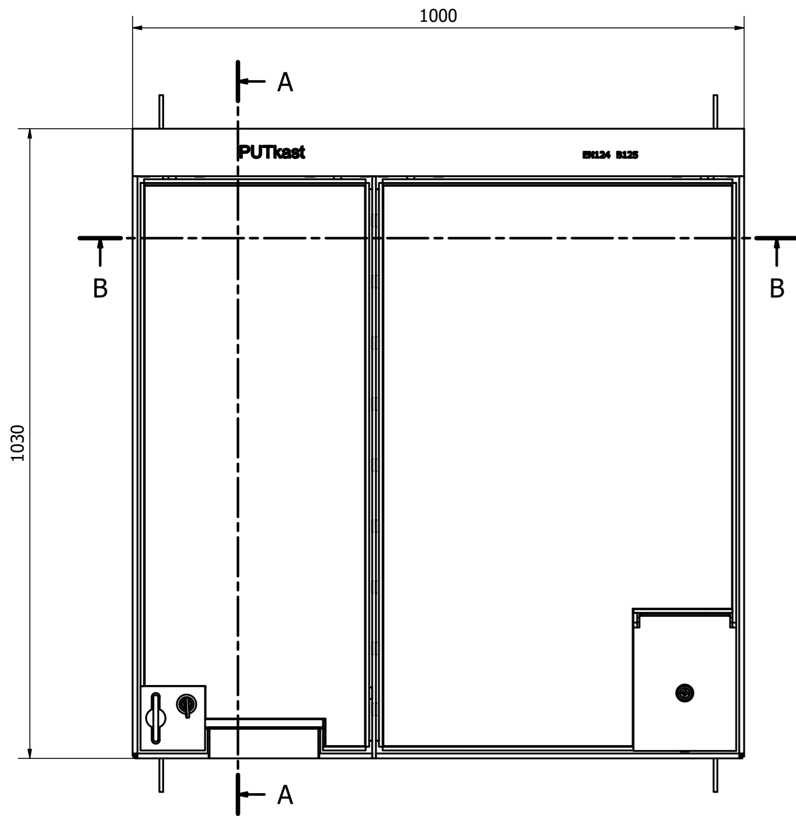
Bovenaanzicht
