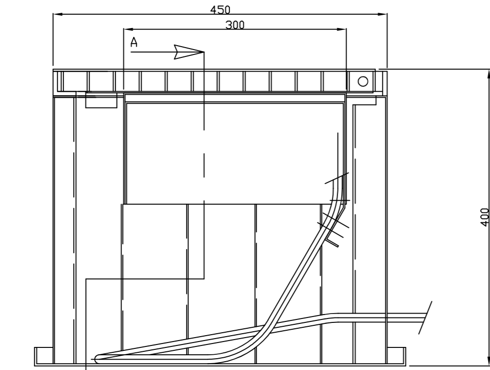
DOORSNEDE B-B
